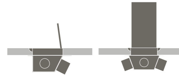
Steckerwanne mit Klappdeckel einseitig und zweiseitig bedienbar, Integration erfolgt direkt in der Tischplatte Power outlet box with hinged lid, can be used from one or both sides, integrated directly into the desk top
